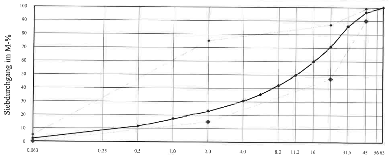
Maschenweite-> | <- Quadratlochweite in mm Sieblinienbereich für Frostschuttschichten 0/45 nach TL SoB-StB 20
